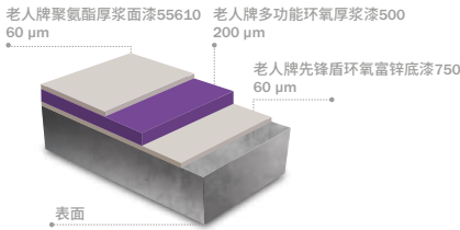
C5 VH - 超过25年 总膜厚320 μm
