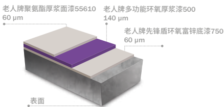
C5 H: 15~25年 总膜厚260 μm
